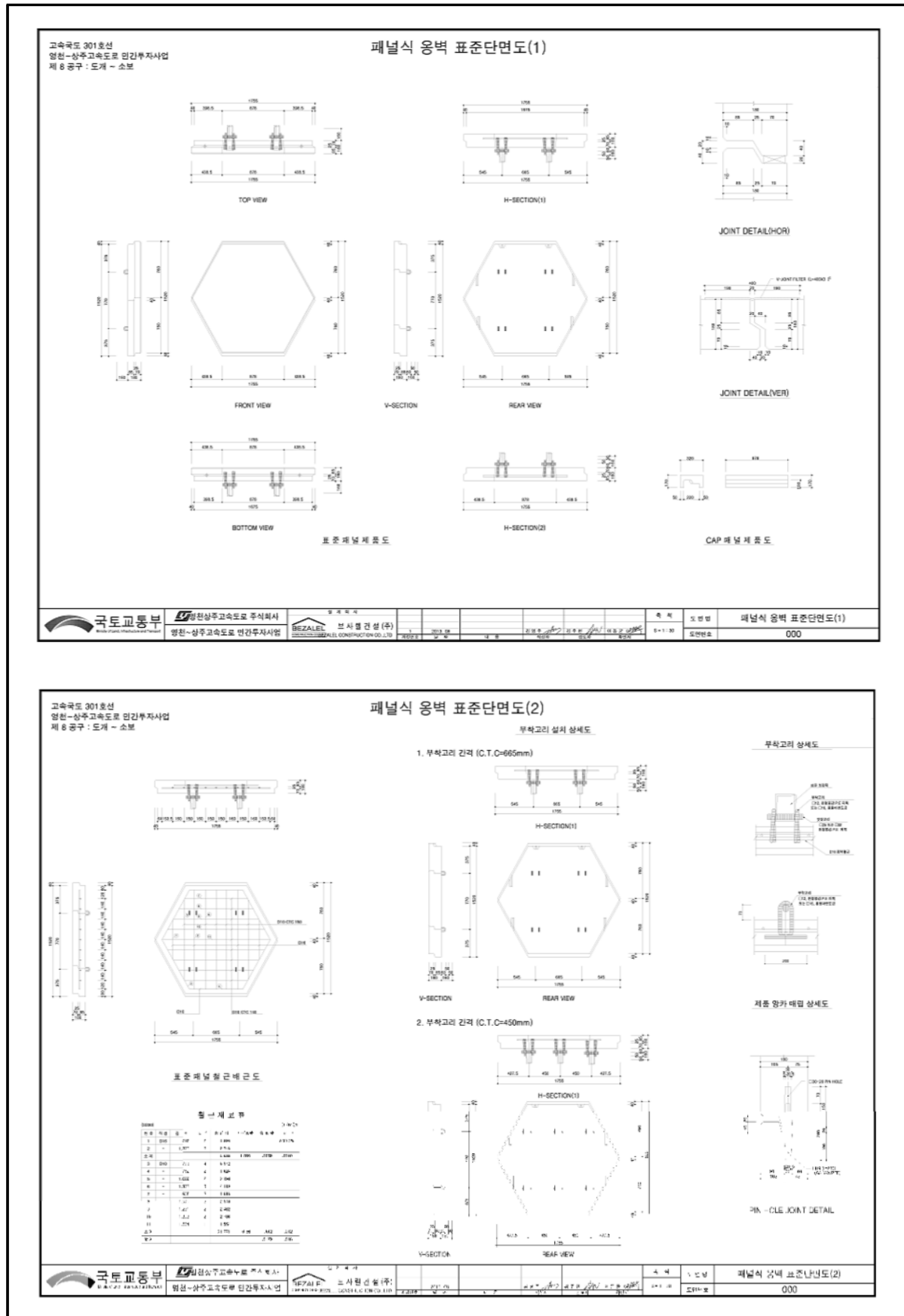
【그림 2.1.4】 단면도
