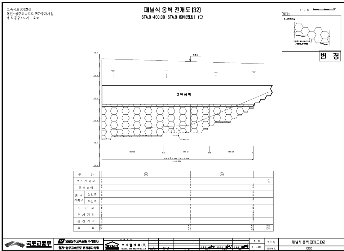
【그림 2.1.3】 전개도(계속)
